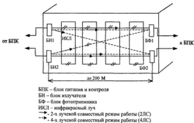
Вариант 2. Блокировка периметра здания извещателем активным оптико-электронным
