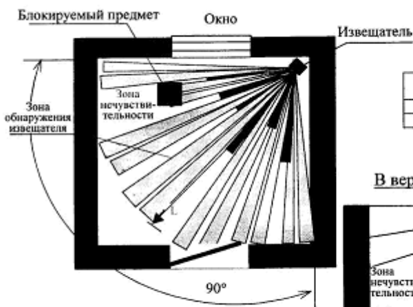
Вариант 7. Одновременная блокировка объема и отдельных предметов оптико-электронным извещателем
