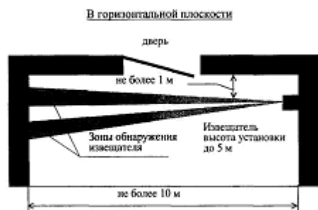
Вариант 4. Блокировка двери на проникновение извещателями магнитоконтактным и поверхностным оптико-электронным с зоной обнаружения типа "занавес"
