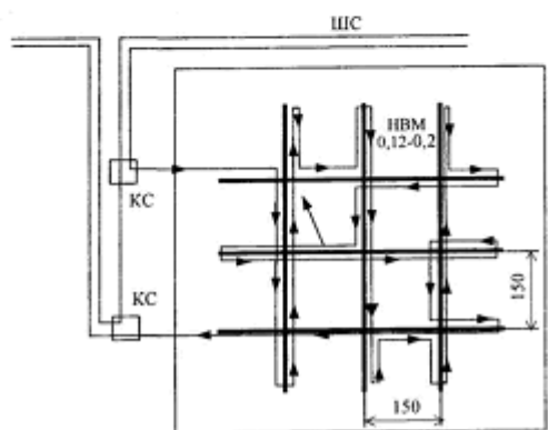
Вариант 2. Блокировка неоткрывающихся решеток проводом
