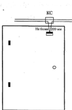
Вариант 2. Блокировка двери на открывание извещателем магнитоконтактным
