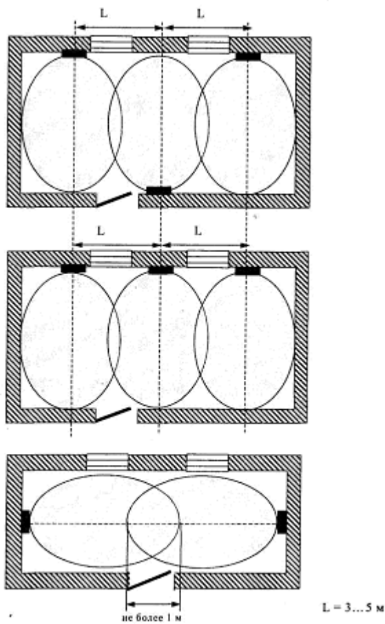
Вариант 2. Блокировка помещения несколькими объемными радиоволновыми (комбинированными) извещателями
