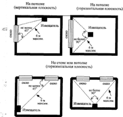
Вариант 6. Блокировка окон (витрин, витражей) на разбитие извещателями поверхностными звуковыми
