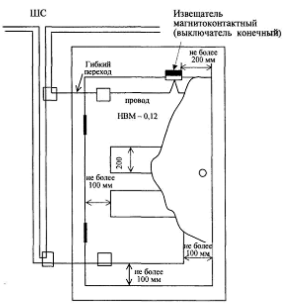
Вариант 1. Блокировка дверей (калиток) на открывание - извещателем магнитоконтактным, на разрушение - проводом
