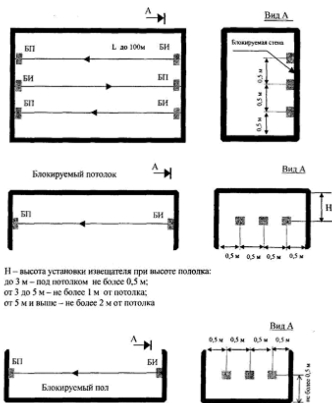
Вариант 5. Блокировка стен, потолка и пола на проникновение извещателями активными линейными оптико-электронными
