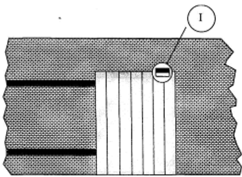
Вариант 2. Блокировка раздвижных ворот выключателем конечным
