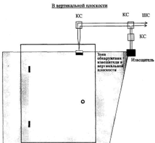
Вариант 3. Блокировка двери на проникновение извещателем поверхностным оптико-электронным с зоной обнаружения типа "занавес"
