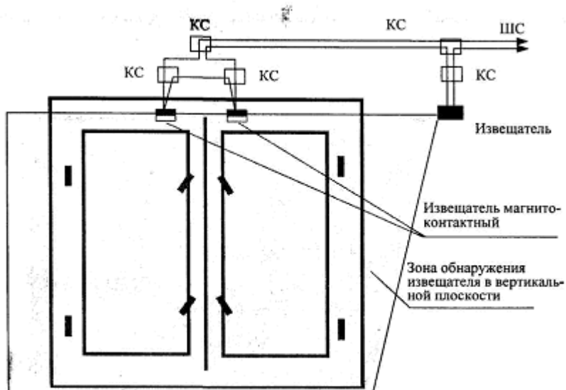
Вариант 4. Блокировка окна на открывание и проникновение извещателем магнито-контактным и поверхностным оптико-электронными с зоной обнаружения типа "занавес"
