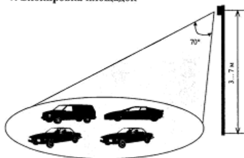
Вариант блокировки открытых площадок ( S, \text{м}^2 = 300...400 ) извещателем объемным радиоволновым
